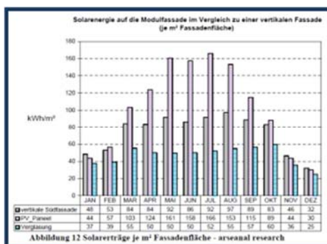
Abbildung 12 Solareträge je m² Fassadenfläche - arseanal research
